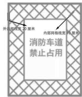
图 2：消防车通道出入口禁停标线及路面警示标志示例
