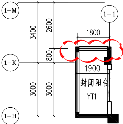
二~二十七层局部平面图 (变更前) 1:100
