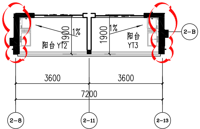
三层局部平面图（变更后） 1:100
