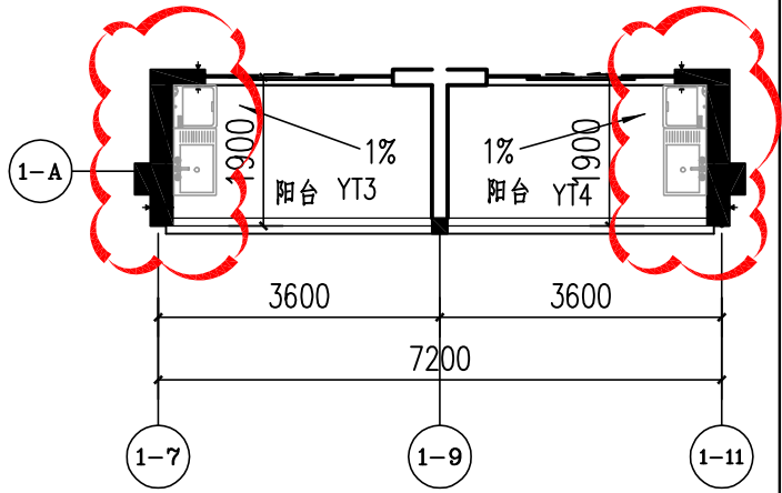
四~十层局部平面图（变更后） 1:100
