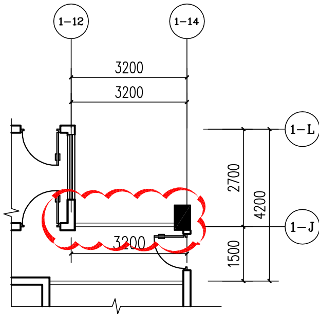
二~二十七层局部平面图 (变更前) 1:100
