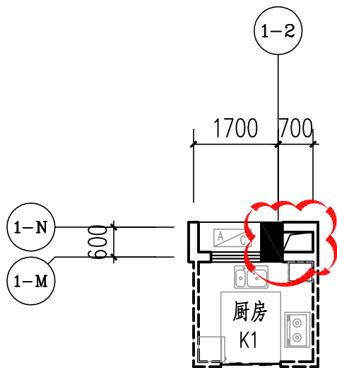
二~二十七层局部平面图（变更前） 1:100
