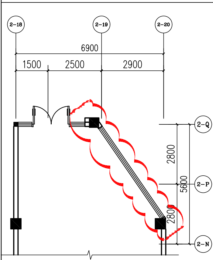
一层局部平面图（变更前） 1:100
