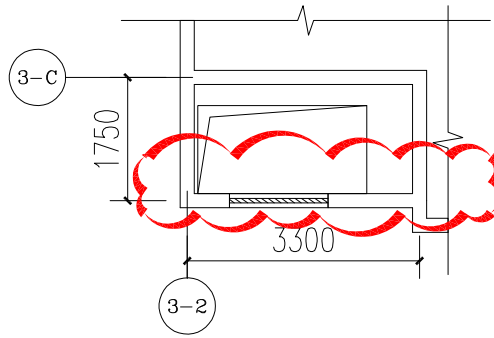
二层局部平面图（变更后）
