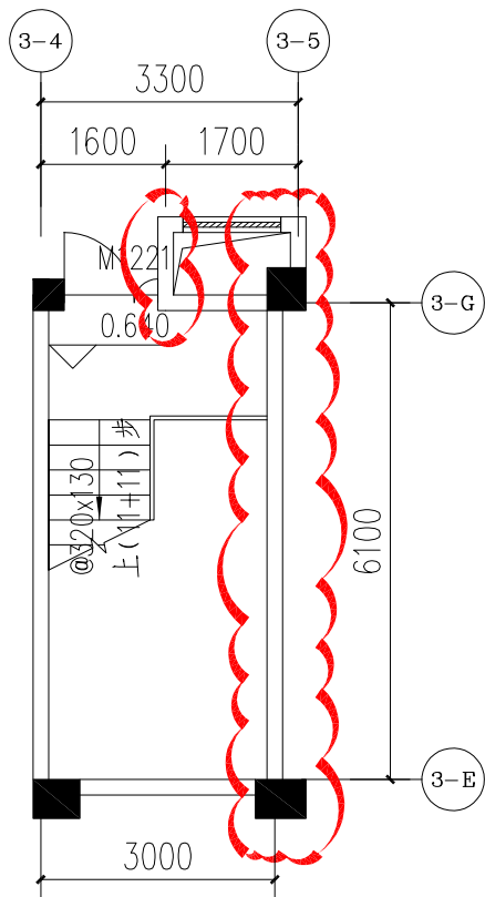
一层局部平面图（变更前）
