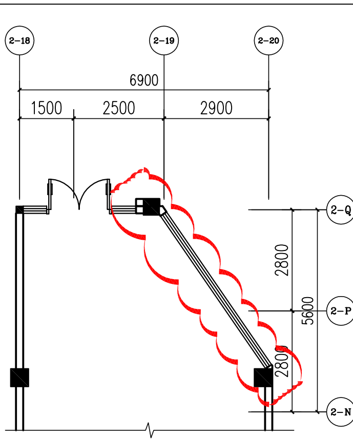
一层局部平面图（变更后） 1:100
