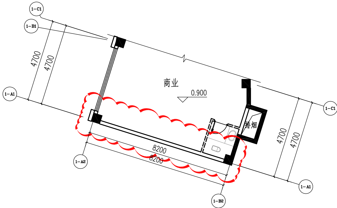
一层局部平面图(变更前) 1:100
