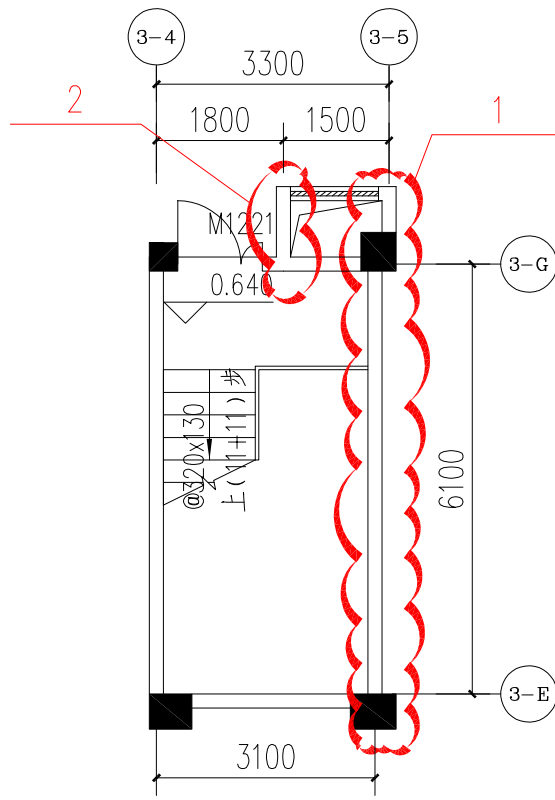
一层局部平面图（变更后）
