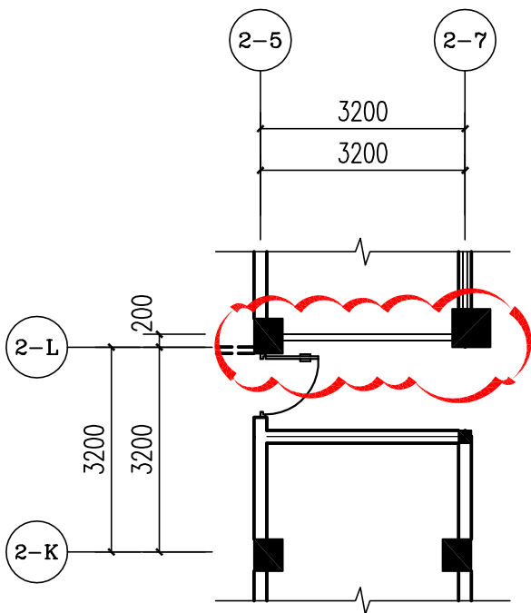
二层局部平面图（变更前） 1:100
