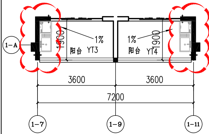
四~十层局部平面图（变更前） 1:100
