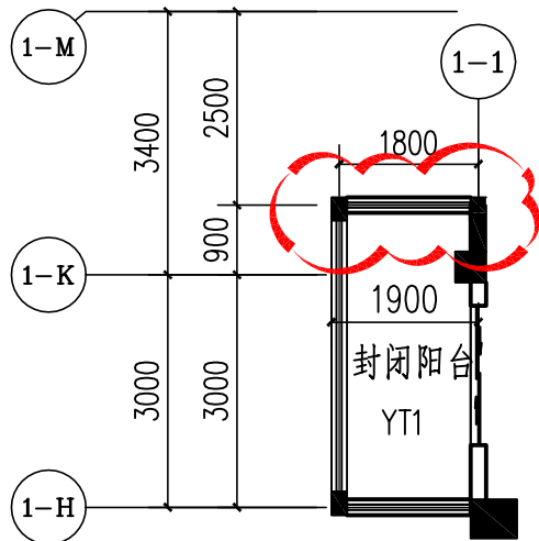
二~二十七层局部平面图 (变更后) 1:100
