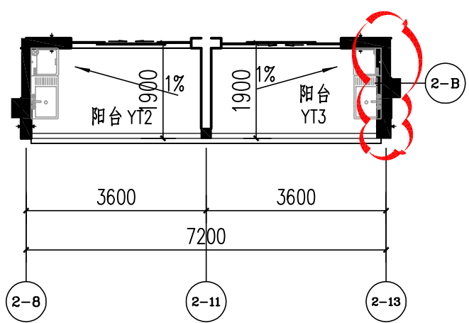
四~七层平面图（变更后） 1:100
