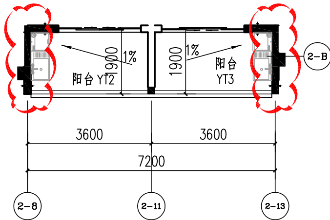
三层局部平面图（变更前） 1:100
