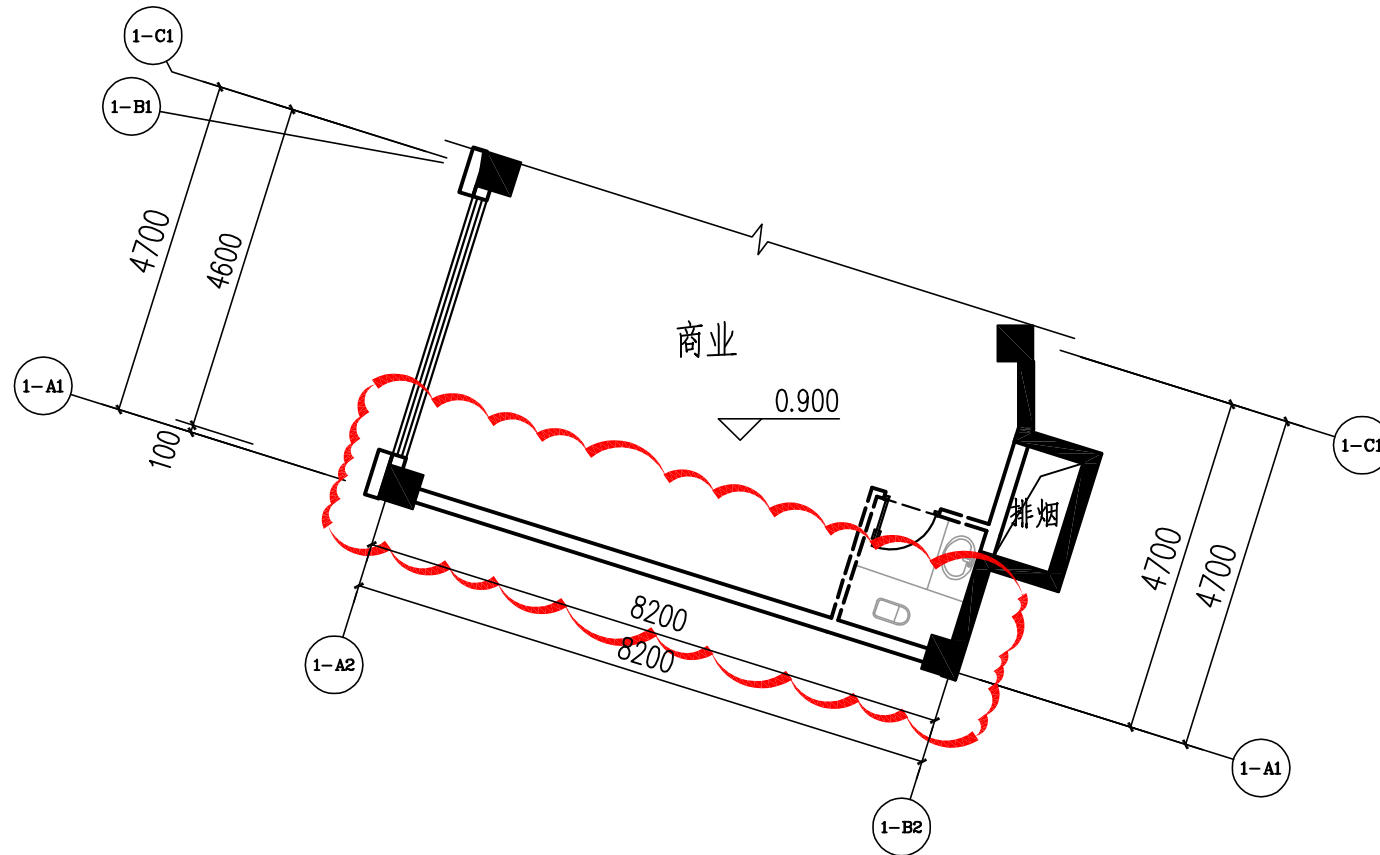
一层局部平面图(变更后) 1:100
