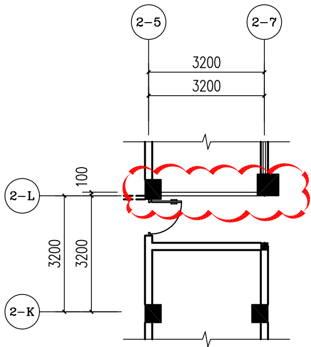
二层局部平面图（变更后） 1:100
