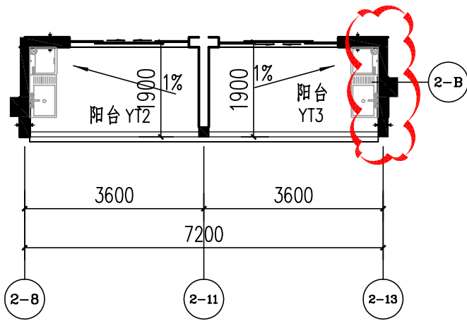
四~七层局部平面图（变更前） 1:100
